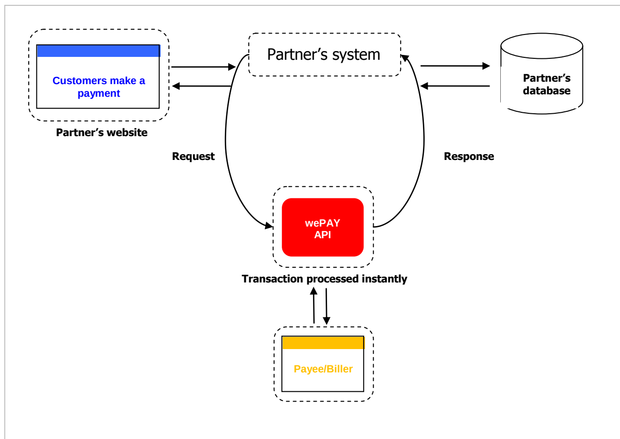
รูปภาพแสดงการทำงานของระบบ wePAY
